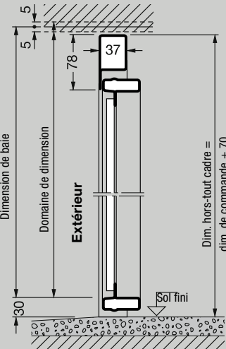
Coupe verticale
