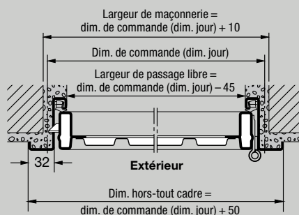
Coupe horizontale
