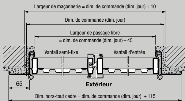
Coupe horizontale
