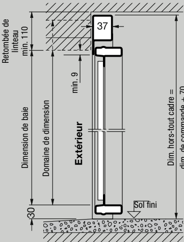
Coupe verticale
