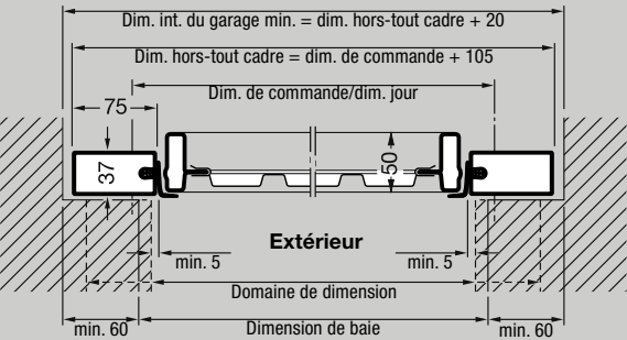
Coupe horizontale
